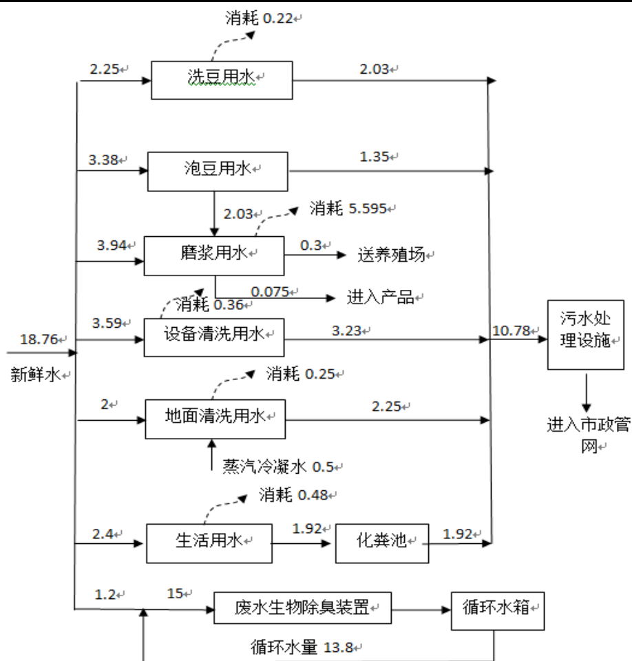
图 2 本项目水平衡图 单位：t/d
