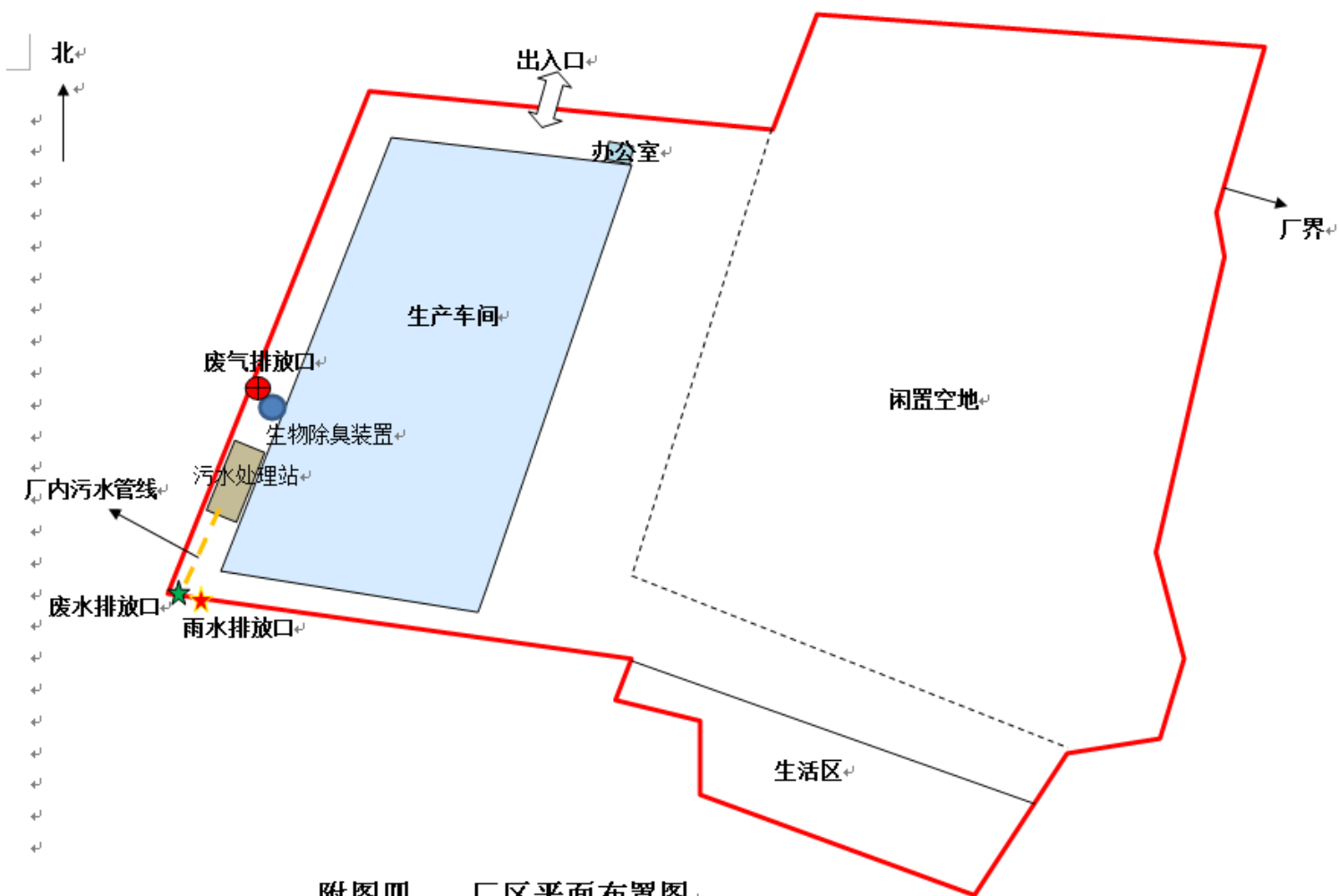
附图四 厂区平面布置图
