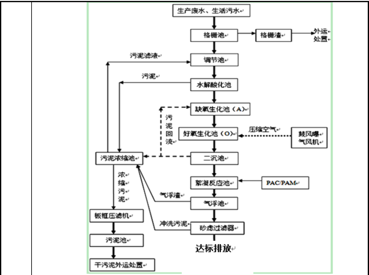
图 4 污水处理工艺流程图
